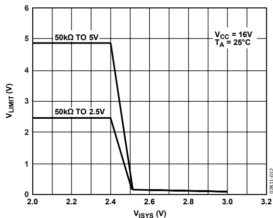
Figure 12. V_{LIMIT} vs. V_{SYS}
