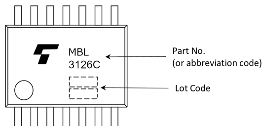
Fig. 6.3 TSSOP14B
