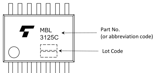
Fig. 6.1 TSSOP14B
