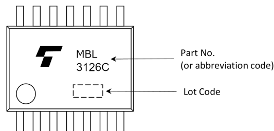
Fig. 6.4 TSSOP14
