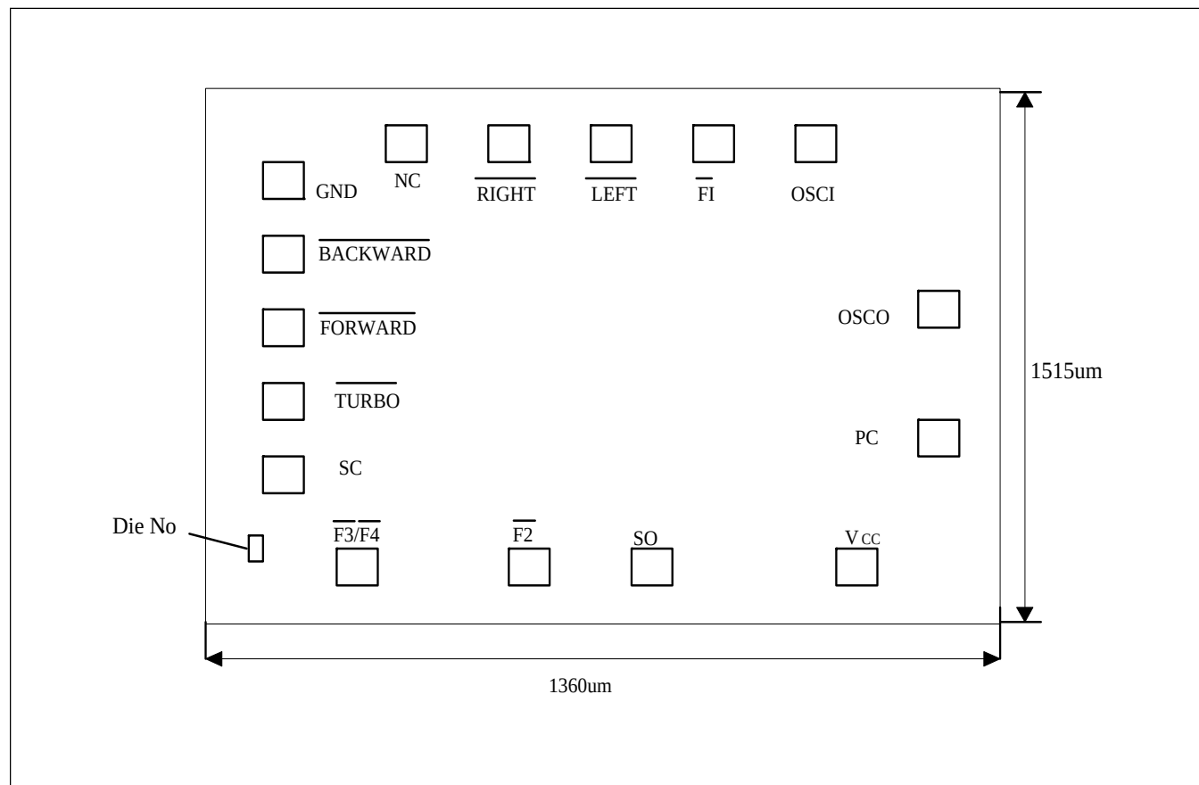
Pad Coordinates
