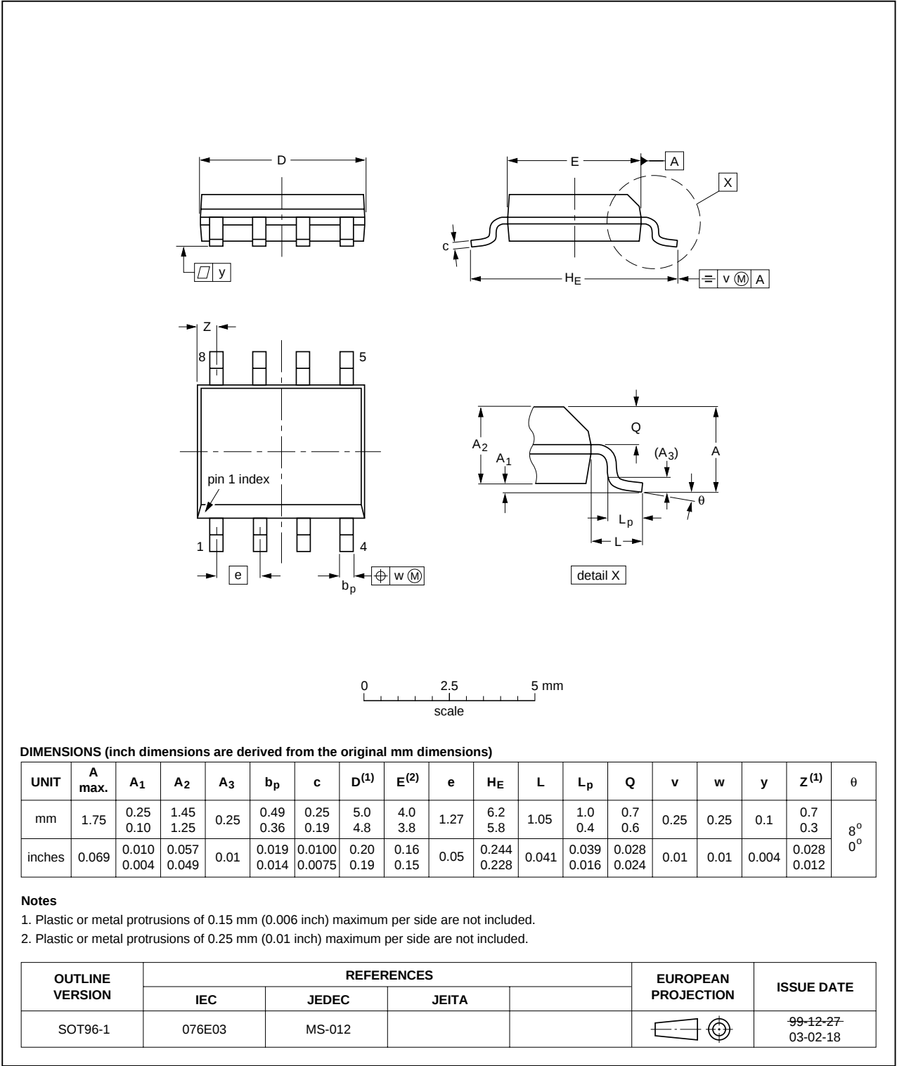
Fig 23. SOT96-1 (SO8).
