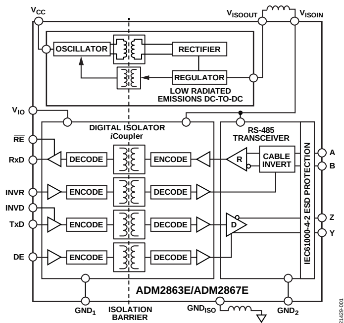
Figure 1. ADM2863E/ADM2867E
