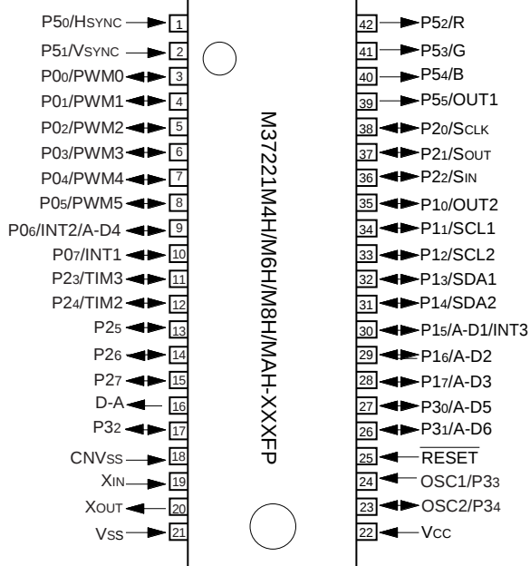
Outline 42P2R-A/E
