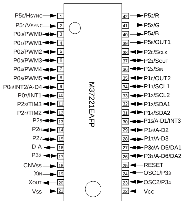
Outline 42P2R-A/E
