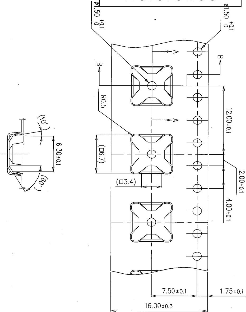
Section A-A
