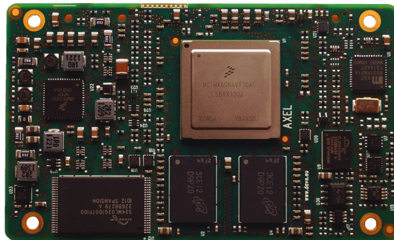
Fig. 2: AXEL SOM (top view)
