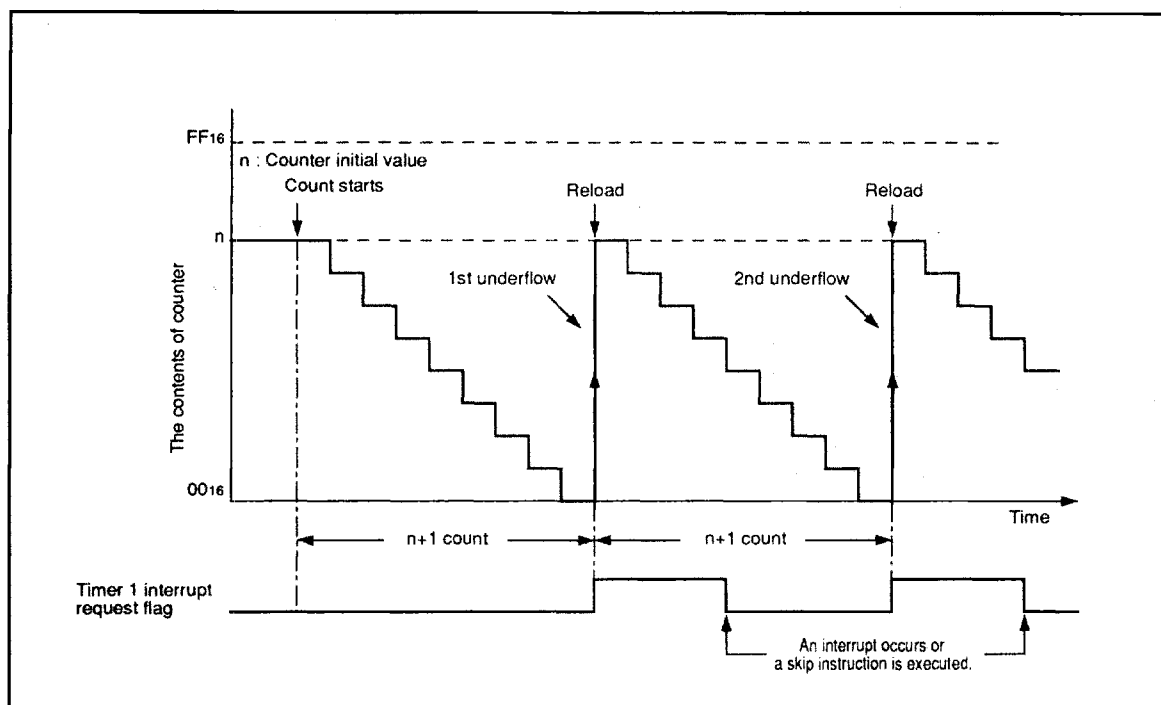
Fig. 20 Auto-reload function
