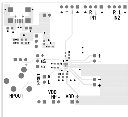
Top Layer
