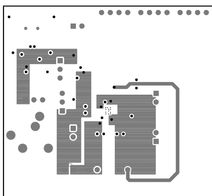
Layer 3
