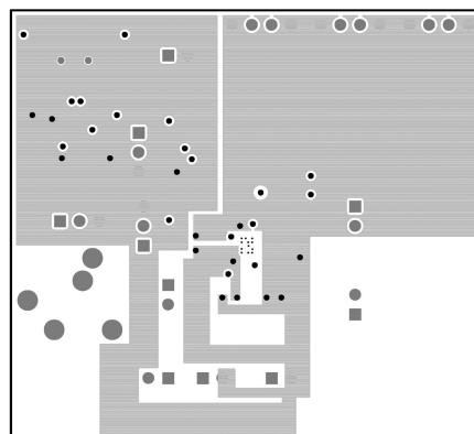
Layer 2
