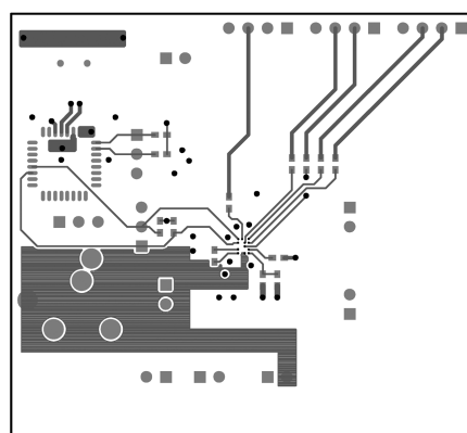
Bottom Layer
