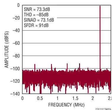
16k Point FFT f_{\text{SMPL}} = 5\text{Msps} , f_{\text{IN}} = 2.2\text{MHz}
