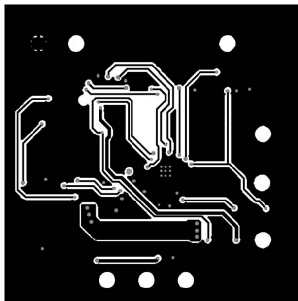
FIGURE 28. BOTTOM LAYER
