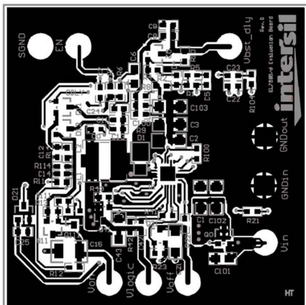
FIGURE 27. TOP LAYER
