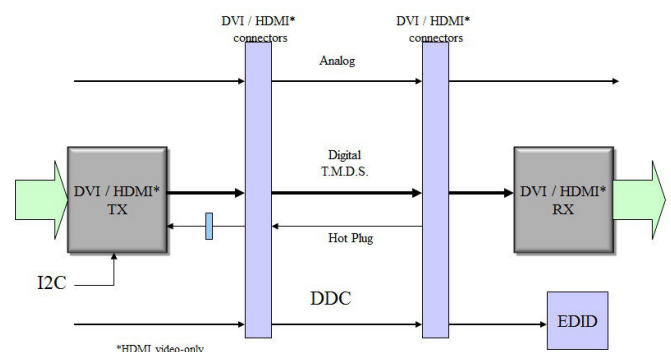
TFP401A-Q1 Diagram
