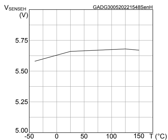
Figure 31. V_{SENSEH} vs T_C
