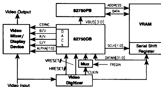
82750DB Subsystem Diagram
