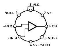
TO-99 (J-Suffix)
