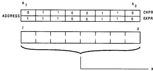
Figure 28. K Parameter Registers (CKPR, EKPR)
