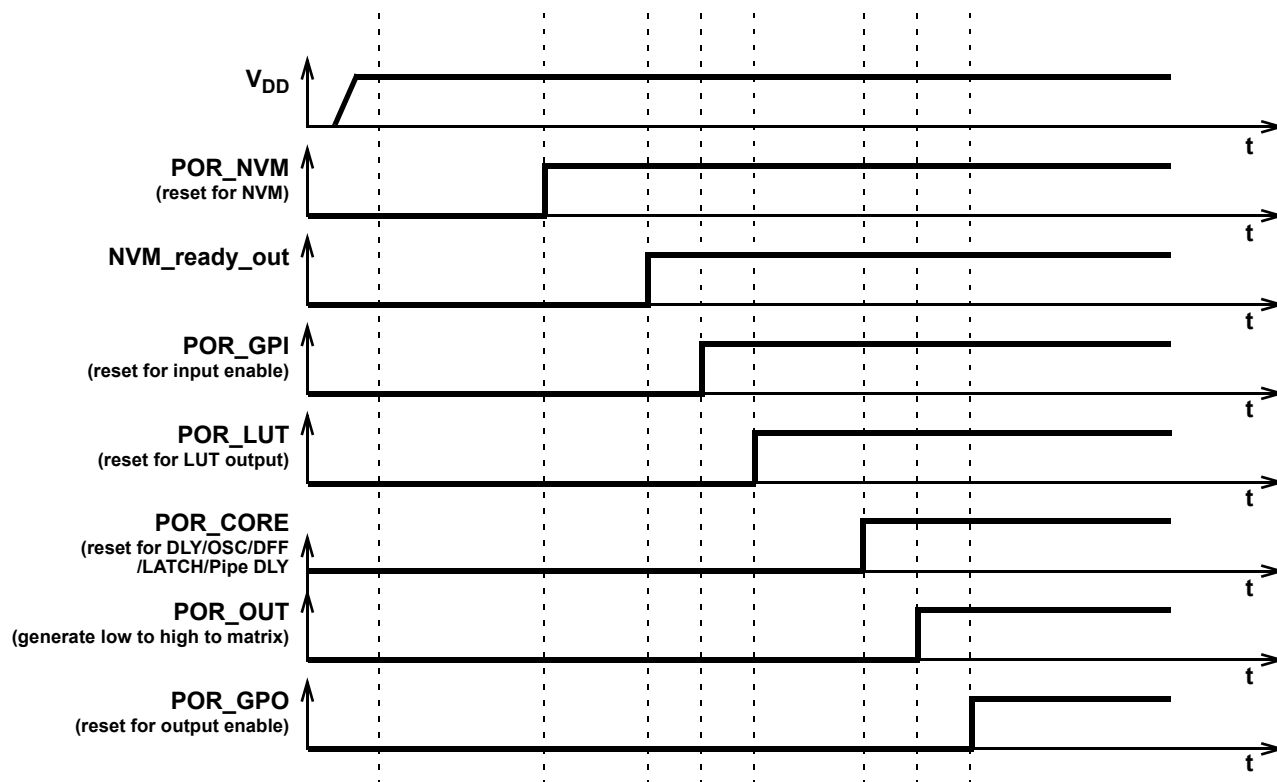
Figure 87: POR Sequence
