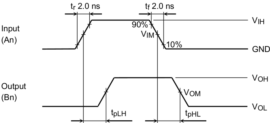
Fig. 12.1 t_{PLH} , t_{PHL}
