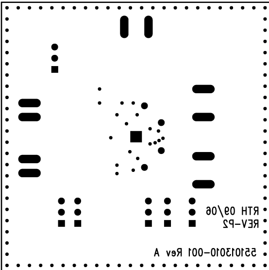
Layer 3
