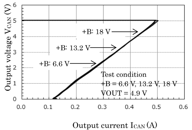
V_{CAN} - I_{CAN}
