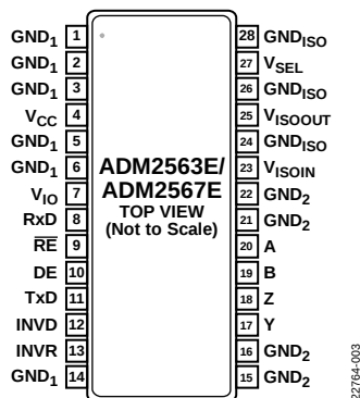
Figure 11. ADM2563E/ADM2567E Pin Configuration
