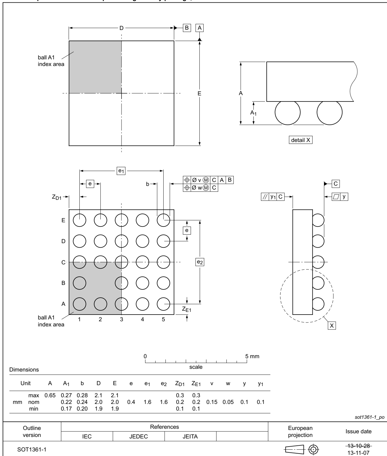
Fig 42. Package outline SOT1361-1 (UFBGA24); ER option
