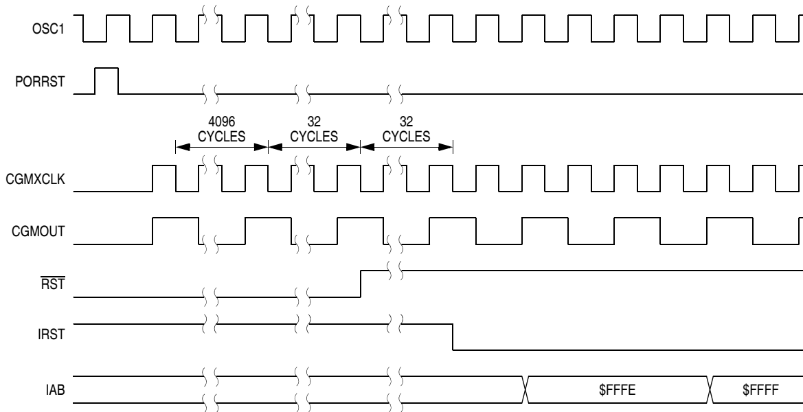
Figure 14-7. POR Recovery
