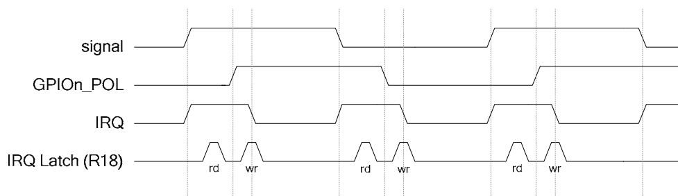
Figure 27 GPIO Edge Detect
