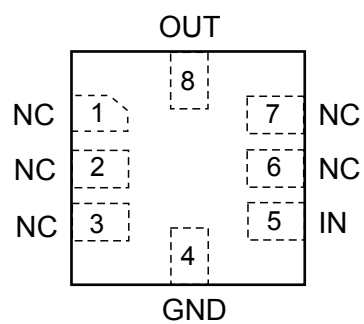
QFN8
