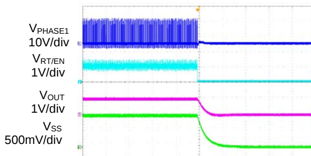
EN Off Waveform
