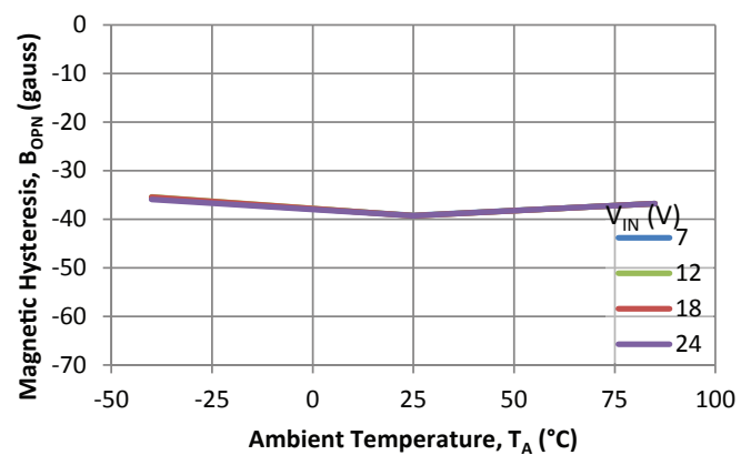
B OPN vs. T A
