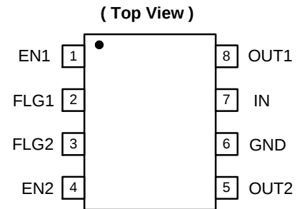
SO-8
