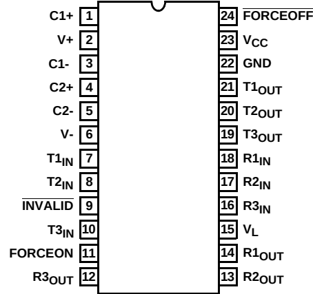
ISL83387E (TSSOP) TOP VIEW
