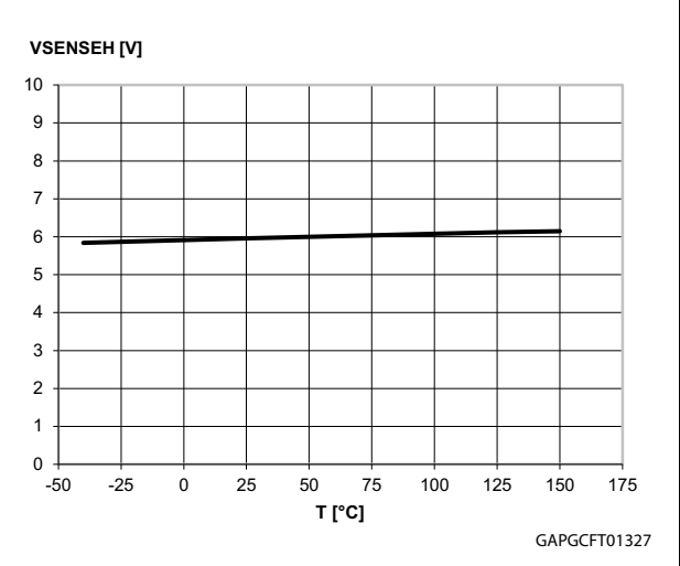
Figure 34. V_{\text{senseh}} vs. T_{\text{case}}
