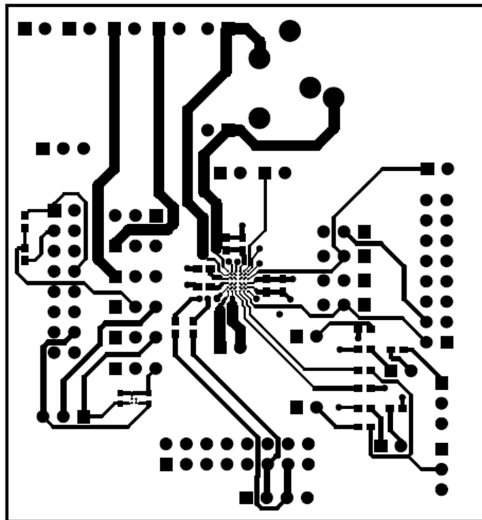
FIGURE 26. Top Layer
