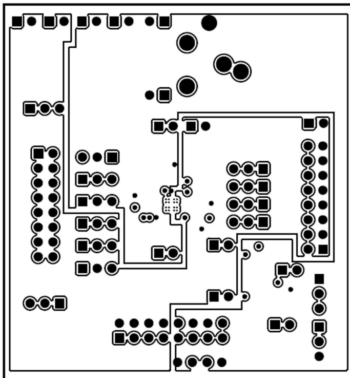
FIGURE 27. Inner Layer 1
