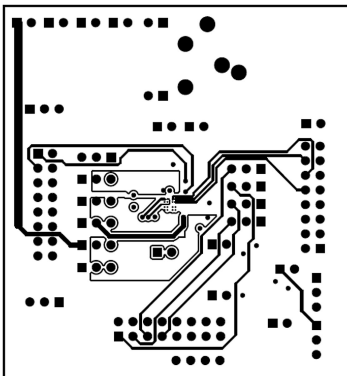
FIGURE 28. Inner Layer 2
