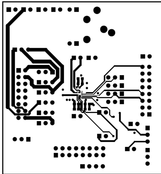
FIGURE 30. Bottom Layer
