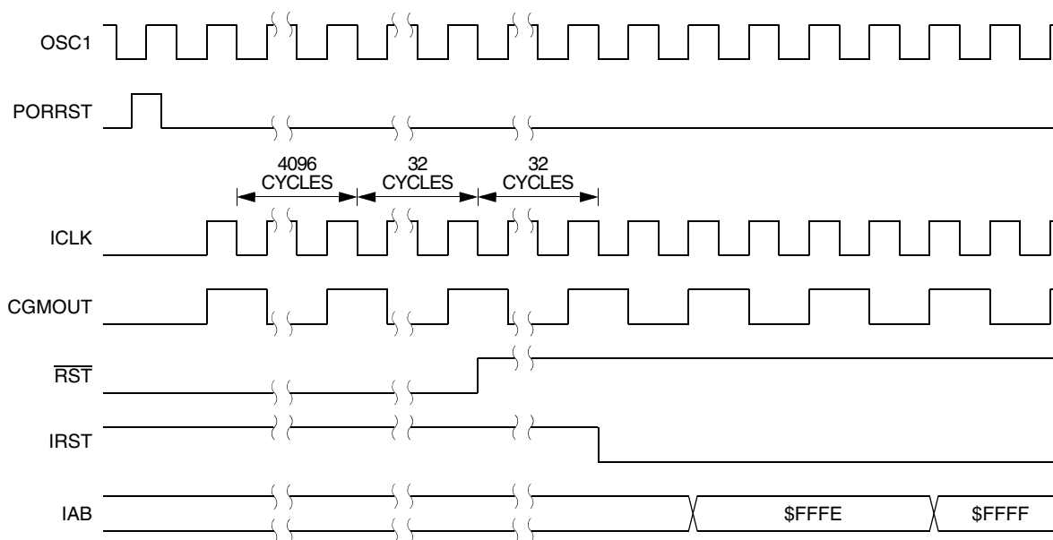
Figure 9-7. POR Recovery
