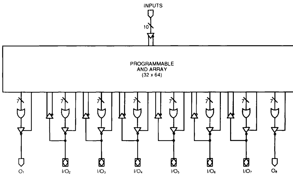
PAL16L8
