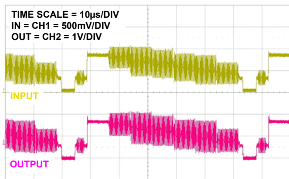
FIGURE 17. NTSC COLORBAR
