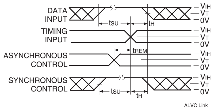
ALVC Link
