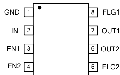
SO-8
