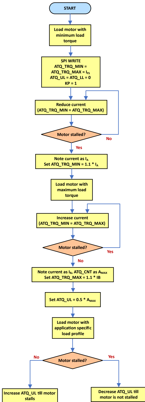
Figure 7-27. Selecting ATQ\_TRQ\_MIN , ATQ\_TRQ\_MAX , ATQ\_UL , ATQ\_LL
