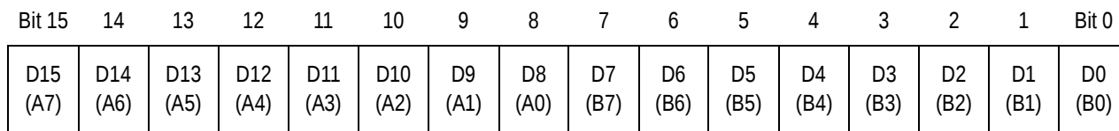
Figure 3-4. Accumulator D (D)
