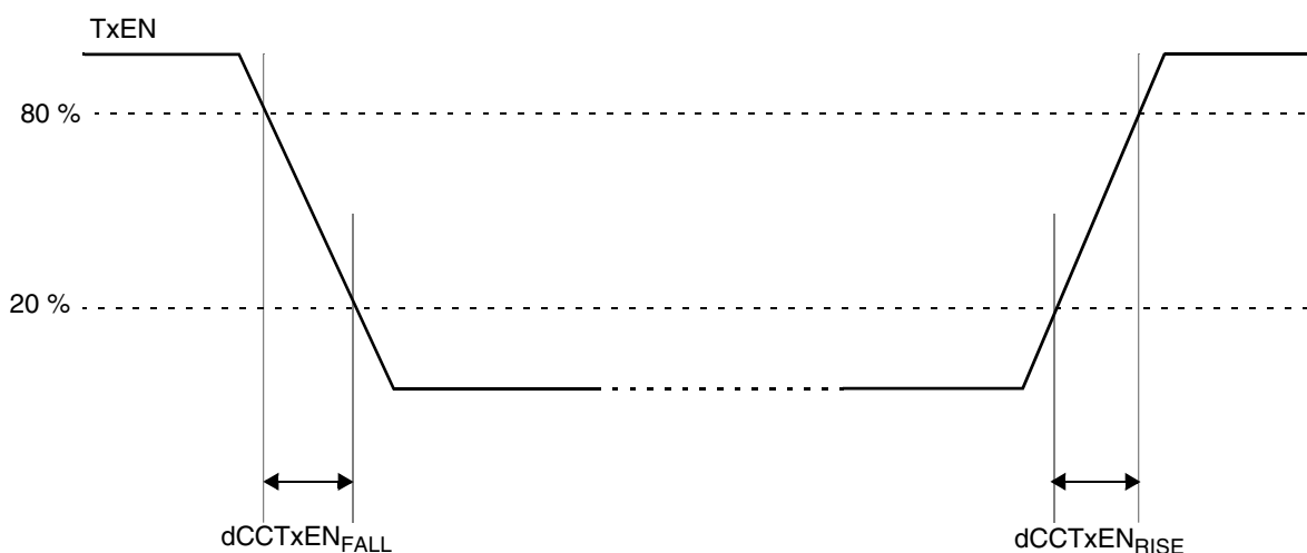
Figure 17. FlexRay TxEN signal
