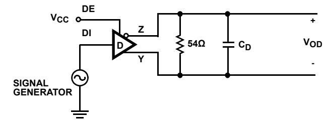
FIGURE 9A. TEST CIRCUIT
