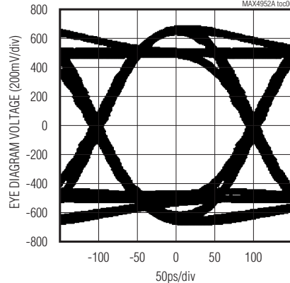
V_{IN} = 275mV_{p-p} , 6Gbps, PE = 1, EQ = 0
