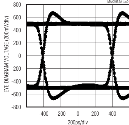
V_{IN} = 275mV_{p-p} , 1.5Gbps, PE = 1, EQ = 0
