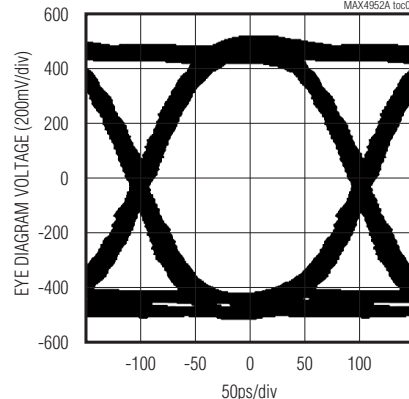
V_{IN} = 275mV_{p-p} , 6Gbps, PE = 0, EQ = 0
