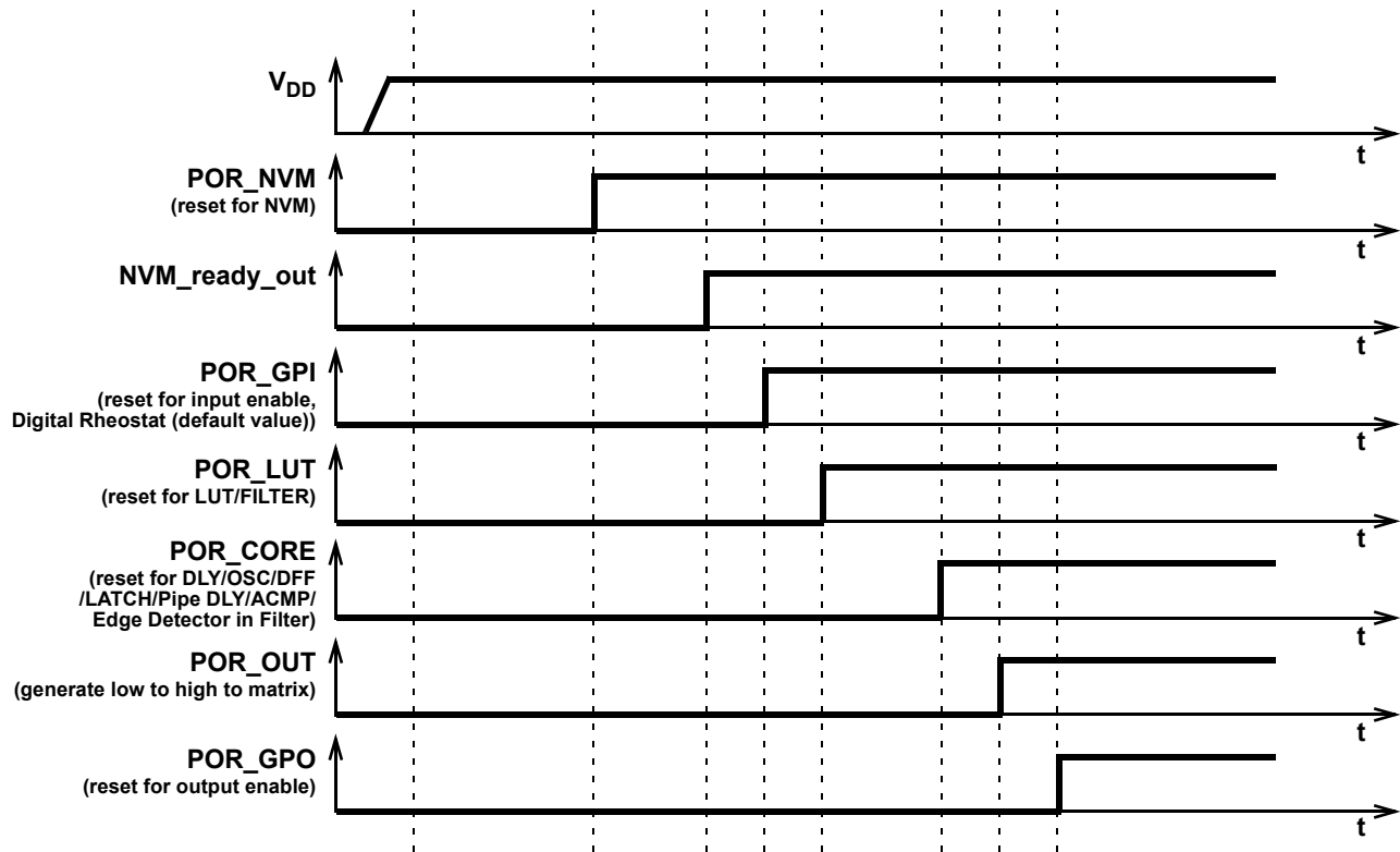
Figure 232: POR Sequence
