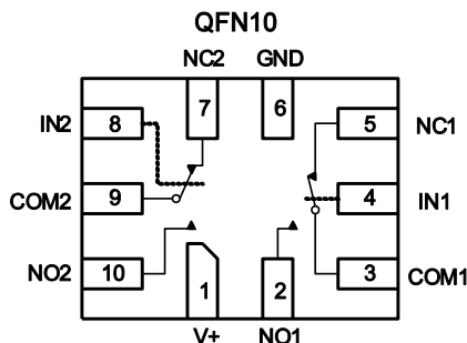
MP2735DQG
