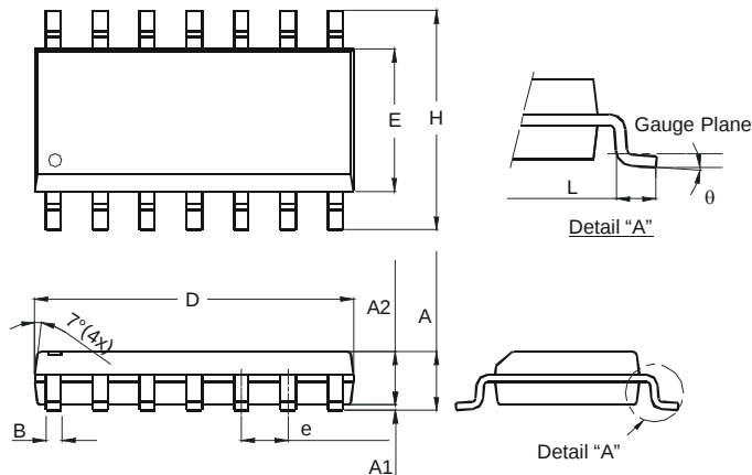
SO-14
