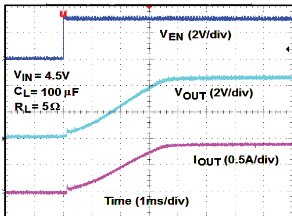
Fig. 22 - Turn-On Time
