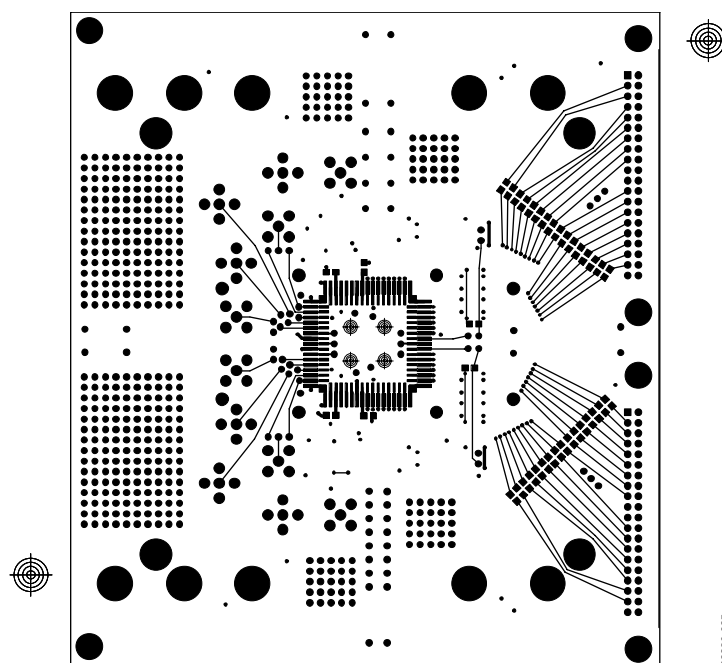
Figure 25. Top Layer
