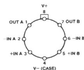
TO-99 (J-Suffix)
