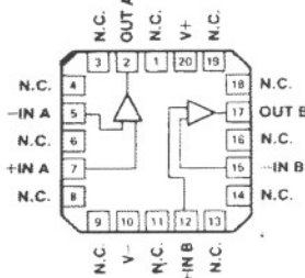
20-CONTACT HERMETIC LCC (RC-Suffix)
