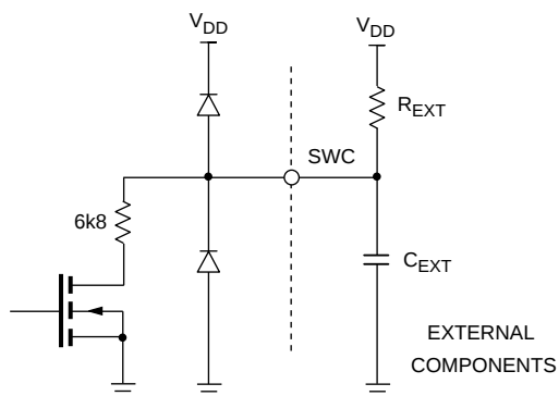
Fig. 5 Pin 15 SWC
