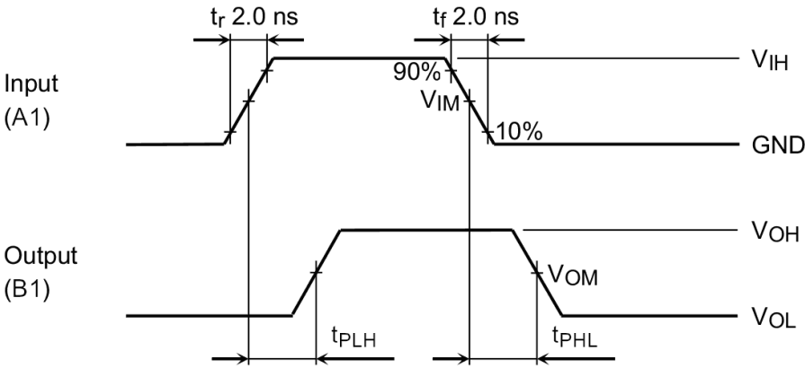
Fig. 13.1 t_{PLH} , t_{PHL}
